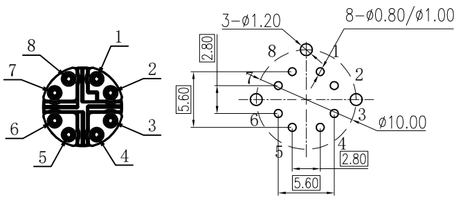
孔位示意图 HOLES ARRANGEMENT
