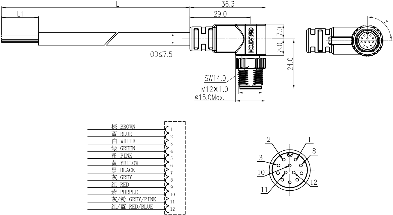
孔位示意图 HOLES ARRANGEMENT
