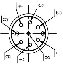
孔位示意图 (8芯) HOLES ARRANGEMENT (8CORE)
